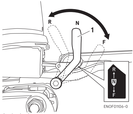
1. Levier inverseur
