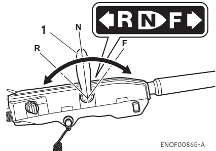
1. Levier inverseur
